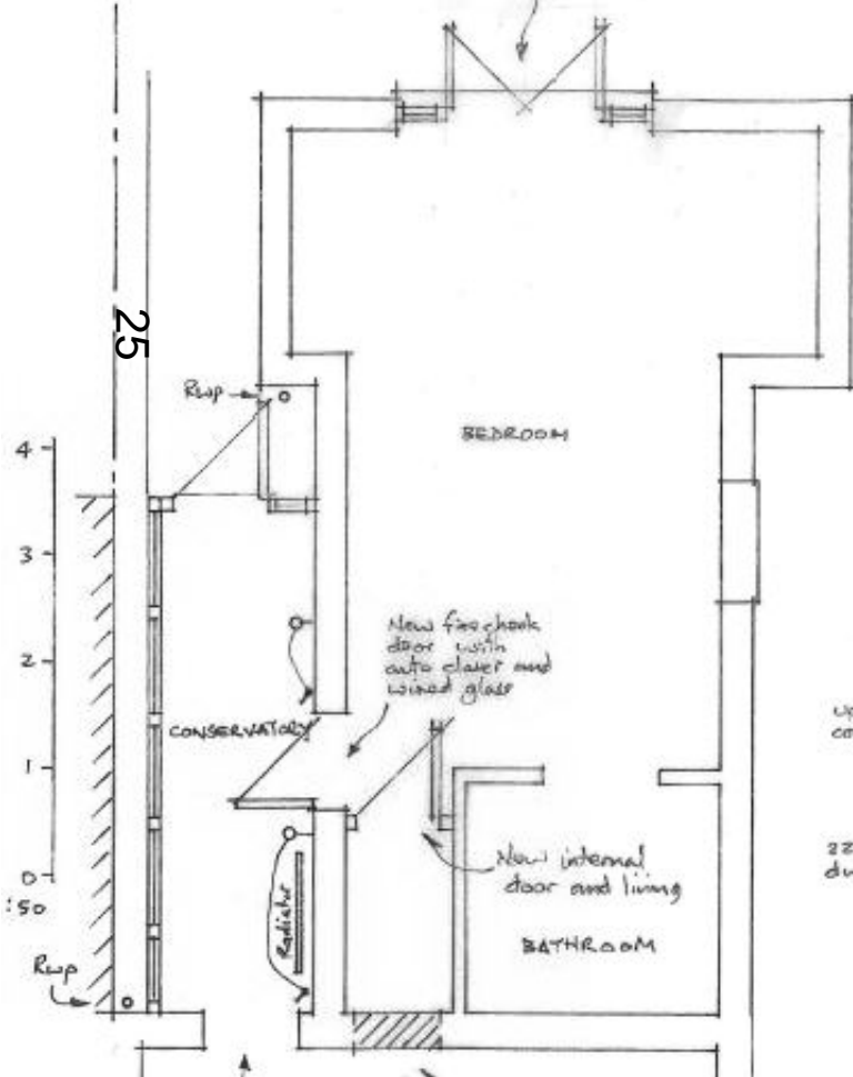
PLAN 1:50
